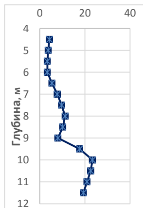
Рисунок 2. – Стратиграфический разрез оз. Кричевичское
