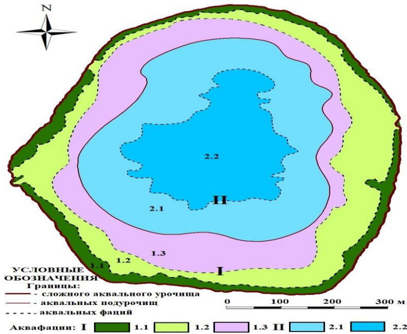
Рисунок 4. – Ландшафтная структура ПАК оз. Кричевичское
