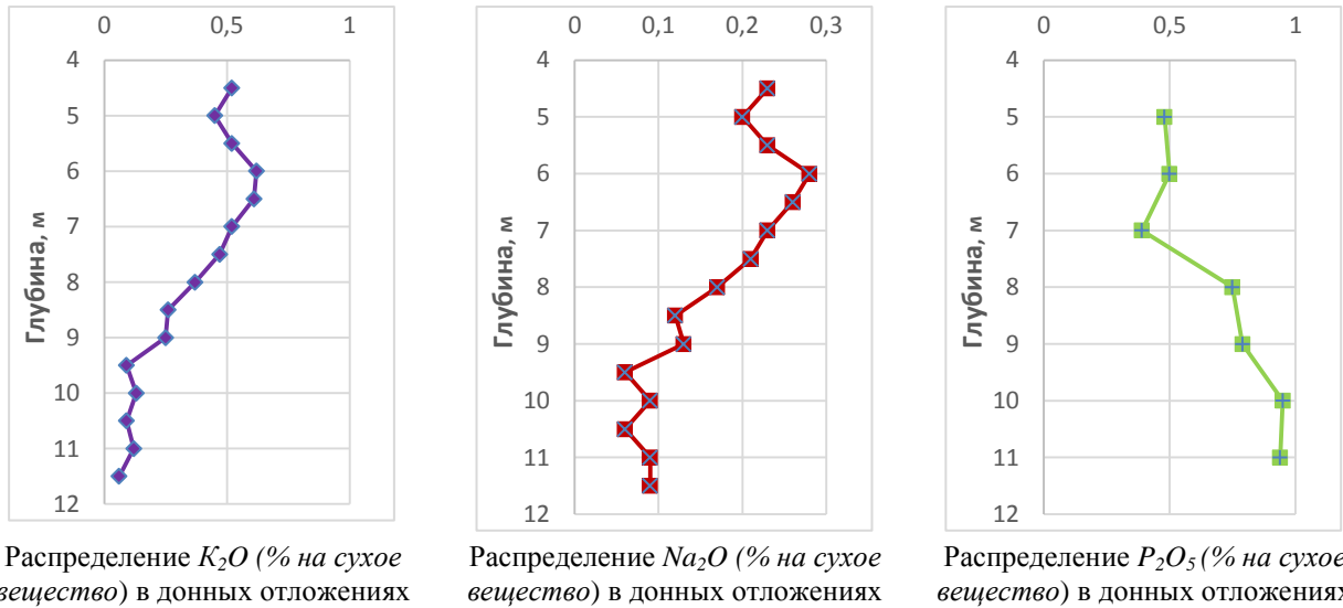
Рисунок 3. – Геохимические особенности донных отложений оз. Кричевичское Примечание – Графики построены по материалам Киевской ГРЭ.
