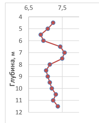
Рисунок 2. – Стратиграфический разрез оз. Кричевичское
